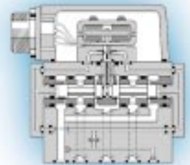
SERVOVALVE
