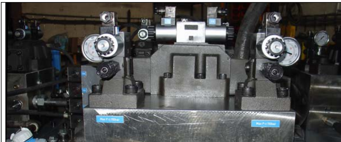
شیر های فشار شکن برقی بلوکی هایدمک
